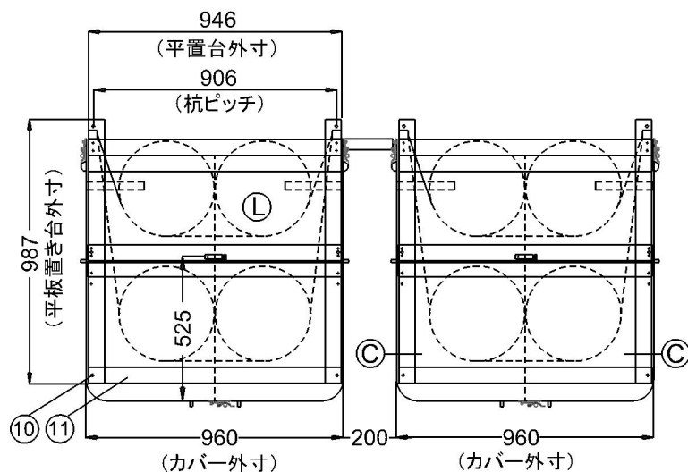
平面
