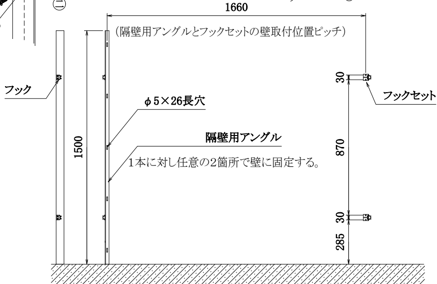
※ 左側面 隔壁用アングル仕様
