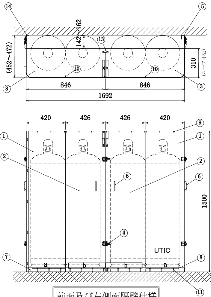
前面及び左側面隔壁仕様
