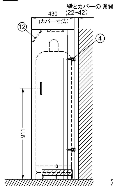
側面
