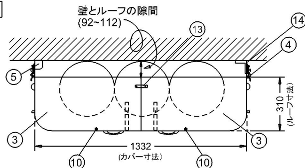
平面
