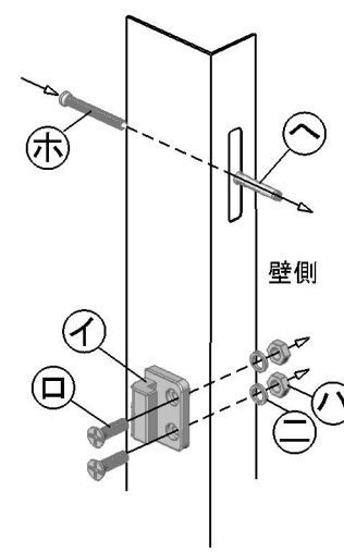
⑭隔壁用アングルセット
