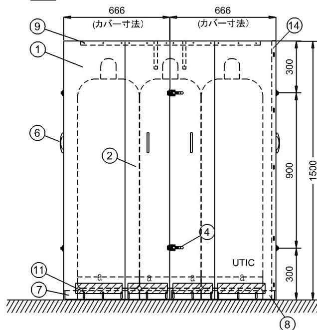
前面
