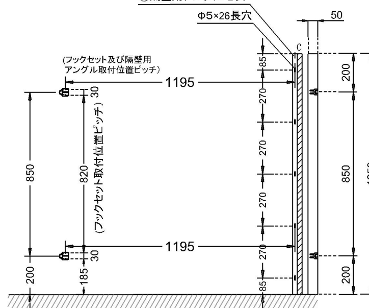
12隔壁用アングルセット
