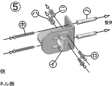
前面及び側面隔壁仕様
