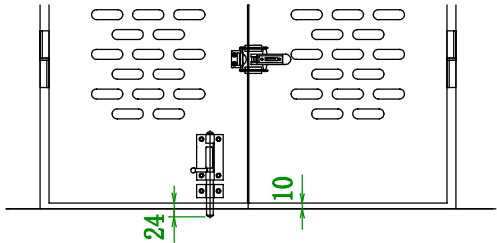
ストローク約44 丸落とし部詳細 丸落とし用ビス M5ナベ×6 M6×15 166個 M6×12 72個
