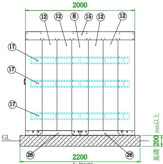
右側面
