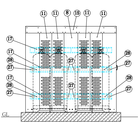
左側面
