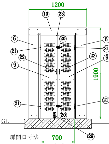
正面
