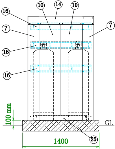
背面
