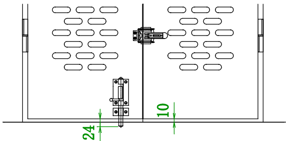
ストローク約44 丸落とし部詳細
