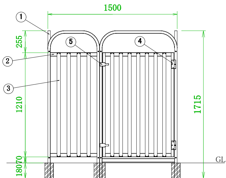
正面図
