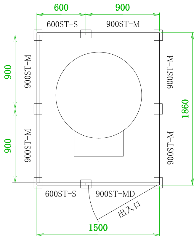
平面図
