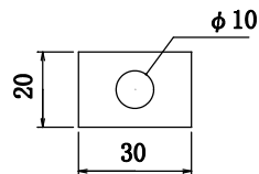
⑰ アルミ製角座金 厚み3
