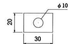
⑮ アルミ製角座金 厚み3
