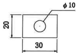
⑮ アルミ製角座金 厚み3
