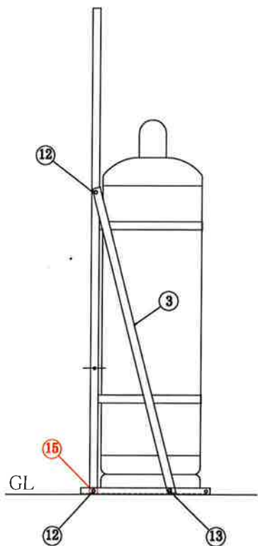
左側面図
