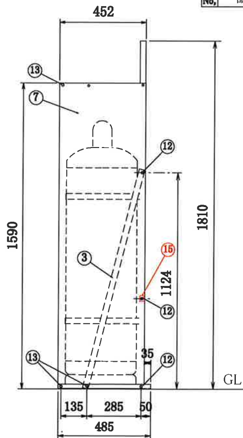
右側面図 (隔壁パネル付 ボンベホルダー) 背面図
