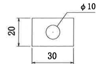
⑮ アルミ製角座金 厚み3
