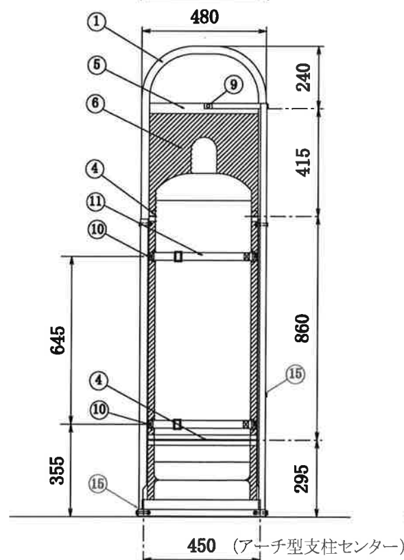
正面図
