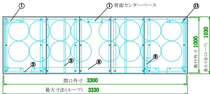
平面
