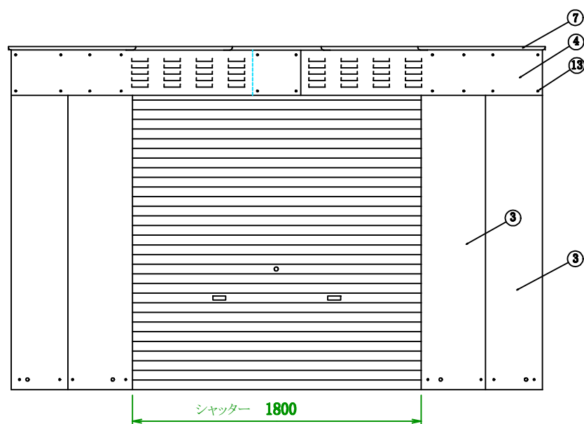
正面
