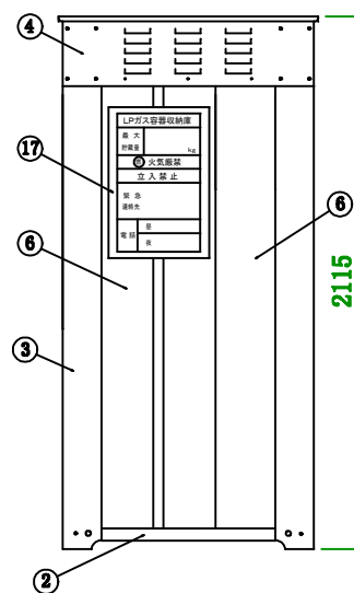
右側面
