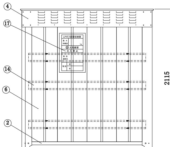
側面図
