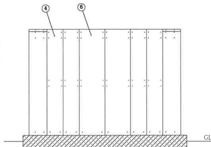
背面
