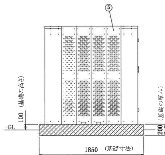
左側面
