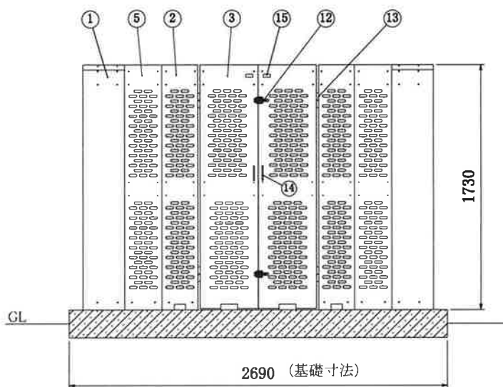
正面
