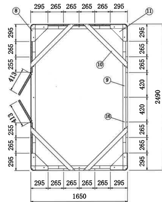
平面
