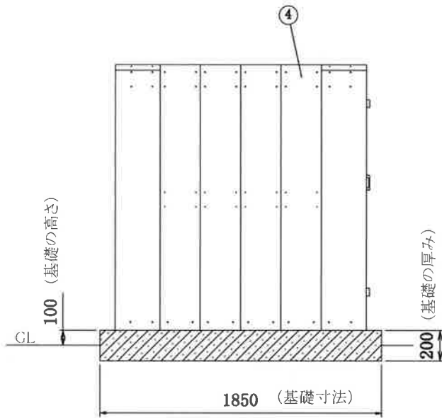
左側面
