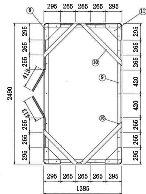
平面
