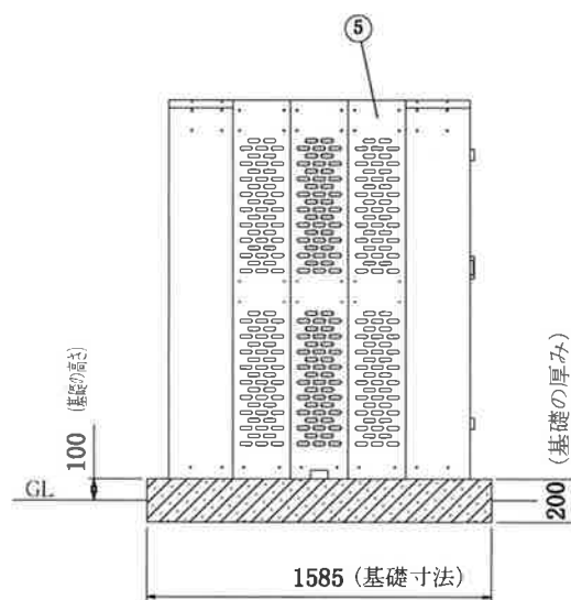
左側面
