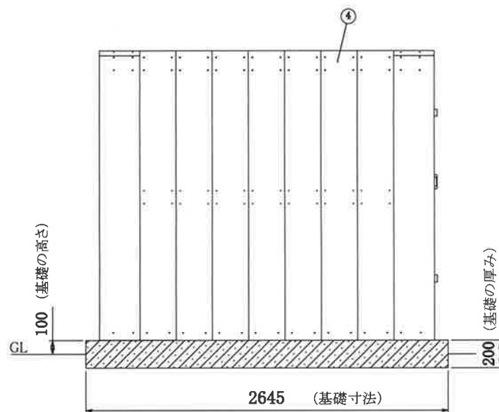
左側面
