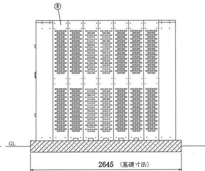
右側面
