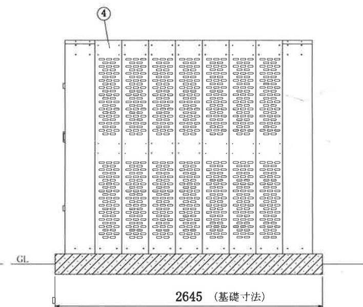
右側面
