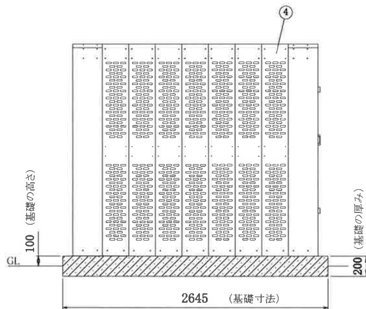
左側面
