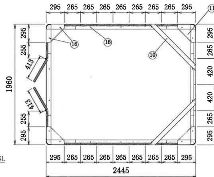
平面
