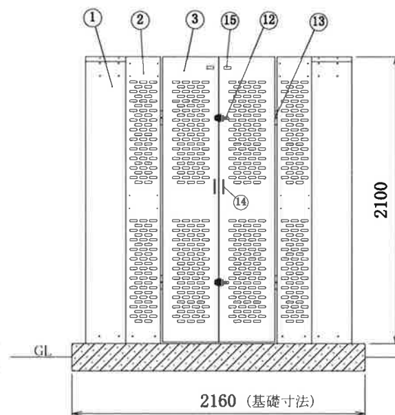
正面
