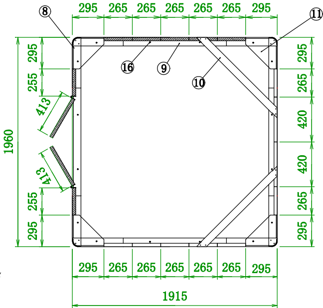
平面
