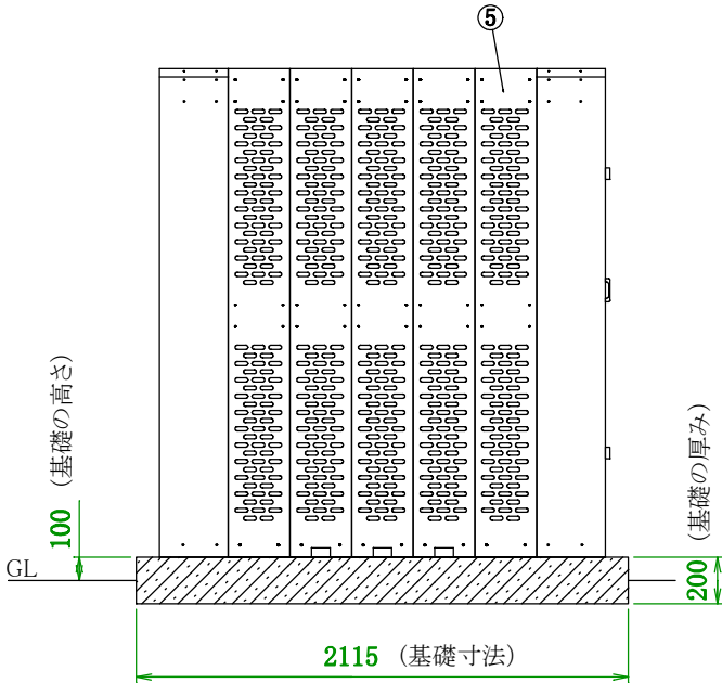
左側面
