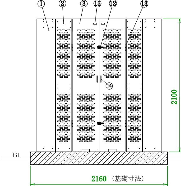
正面
