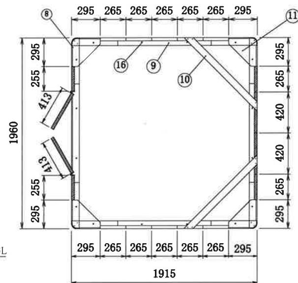
平面
