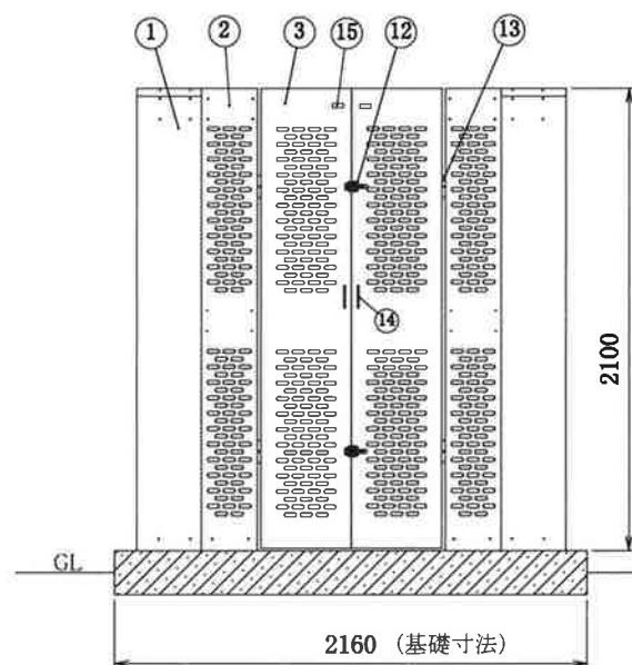
正面
