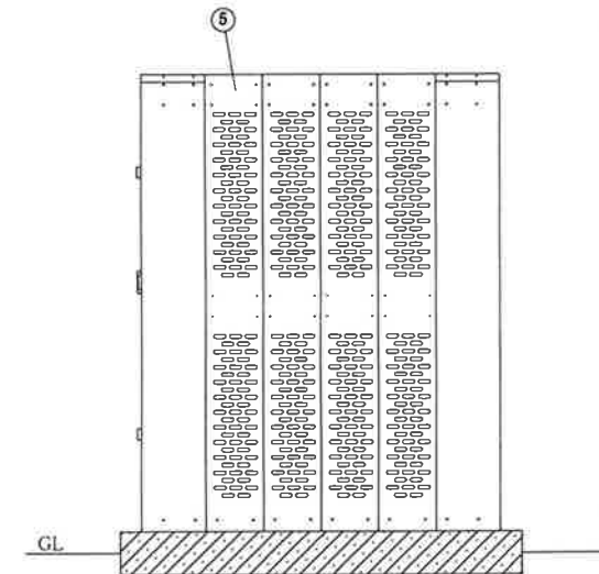
右側面
