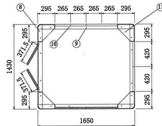
平面
