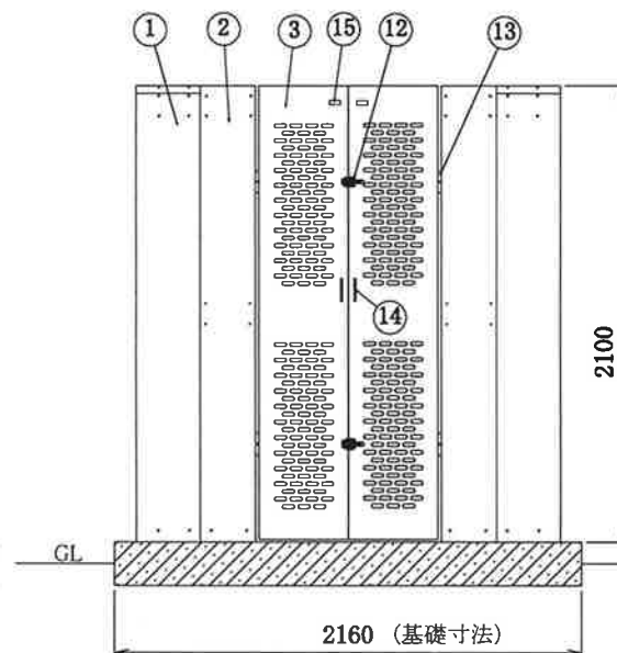
正面
