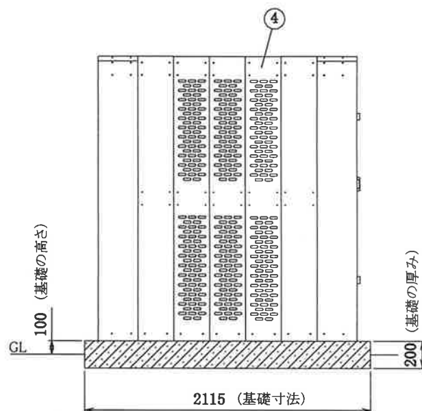
左側面
