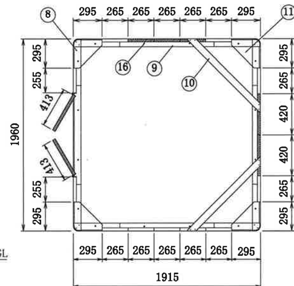
平面
