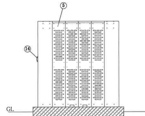
右側面
