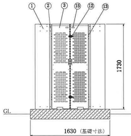
正面
