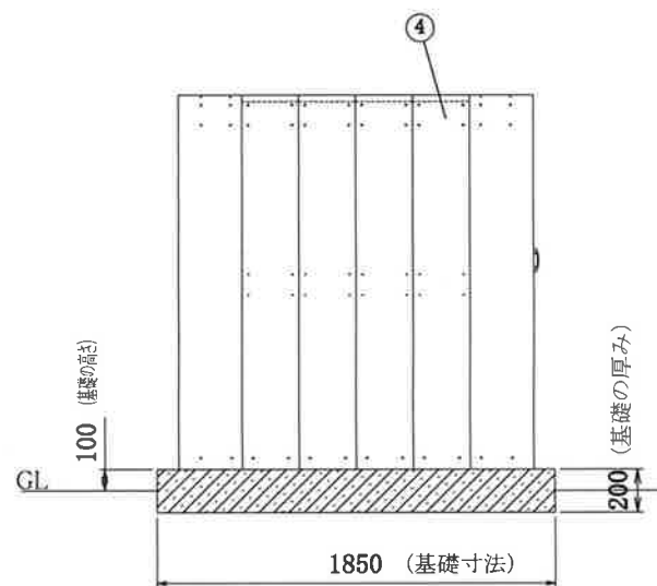
左側面
