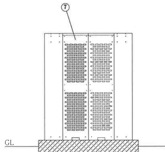
背面
