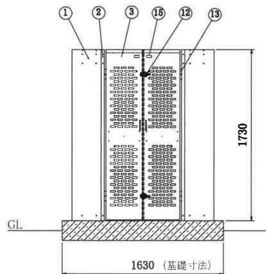
正面
