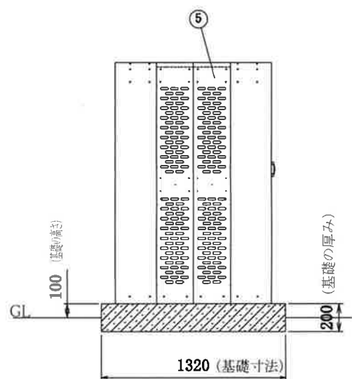
左側面
