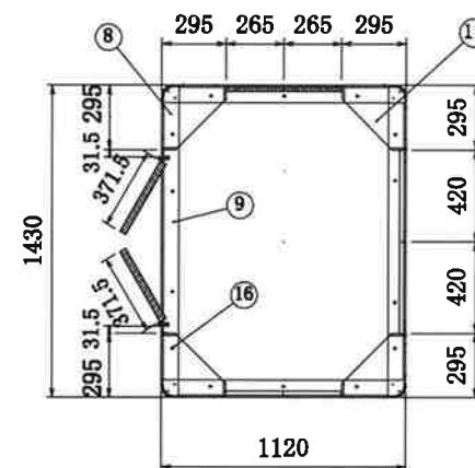
平面
